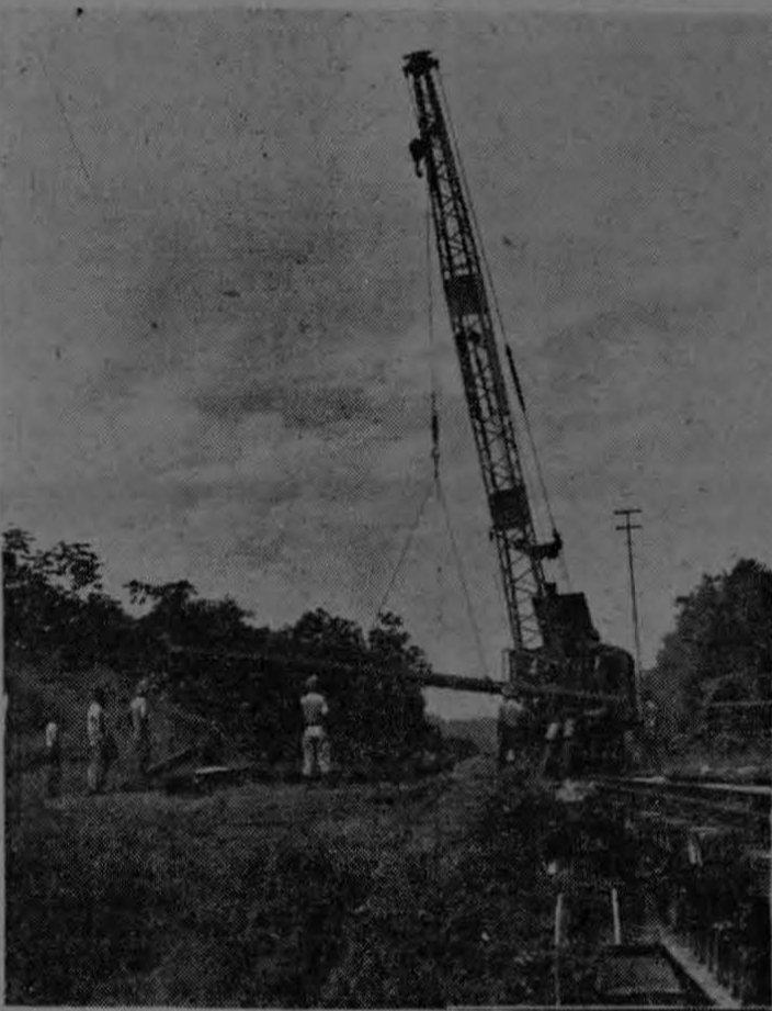
Una potente grúa levanta uno de los largueros que soportarán un nuevo puente en el Valle de Coto. Esta nueva vía, habilitará la región en que se forman los dos nuevos centros de producción: Fincas 54 y 55 de Coto.
